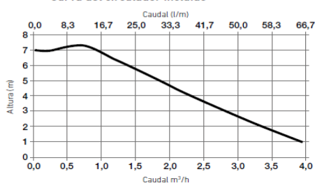
Curva del circulador incluido
